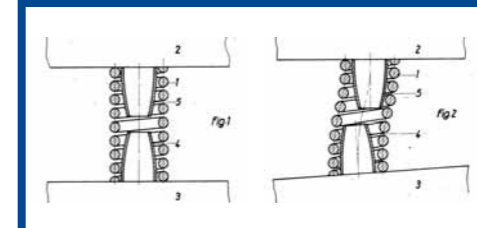
Federn gerade (links), ausgelenkt und geneigt (rechts). Abb. mit Ausknicksicherung, Patent Rhein Stahl-Henschel
