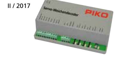
II / 2017 55274 59,99 €* Servo-Weichendecoder Zum digitalen oder analogen Betrieb des Unterflur-Weichenantrieb #55272. Es können bis zu vier Weichenantriebe angeschlossen werden.
