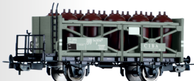
Säuretopfwagen „CIBA AG“, eingestellt bei den SBB Acid pot car „CIBA AG“ of the SBB
